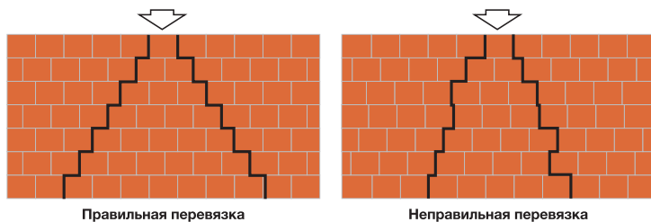
Рис. 10. Примеры перевязки
