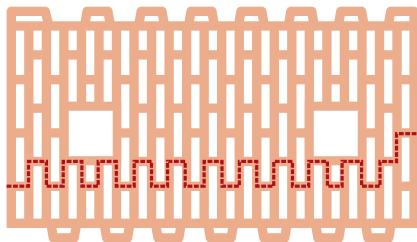
Рис. 5. Теплопередача через керамические стенки
