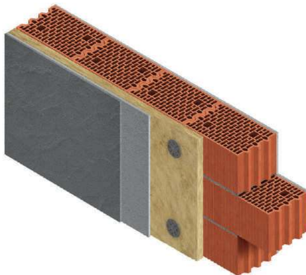
Рис. 3. Конструкция стены из блоков Porothem 25, минераловатных плит и штукатурки
