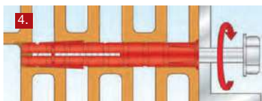
4. Заворачивание шурупа
