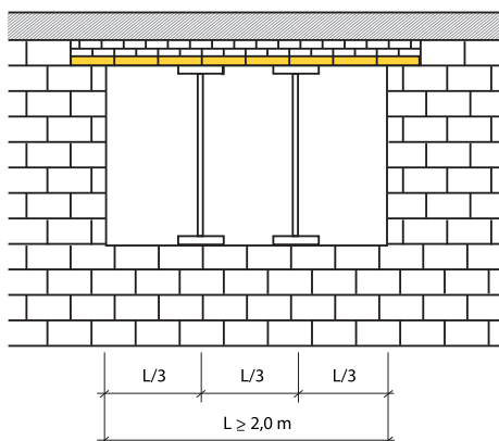
Схема установки подпорной стойки под перемычки длиной свыше 2,0 м
