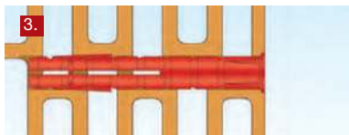
3. Вставка дюбеля в отверстие
