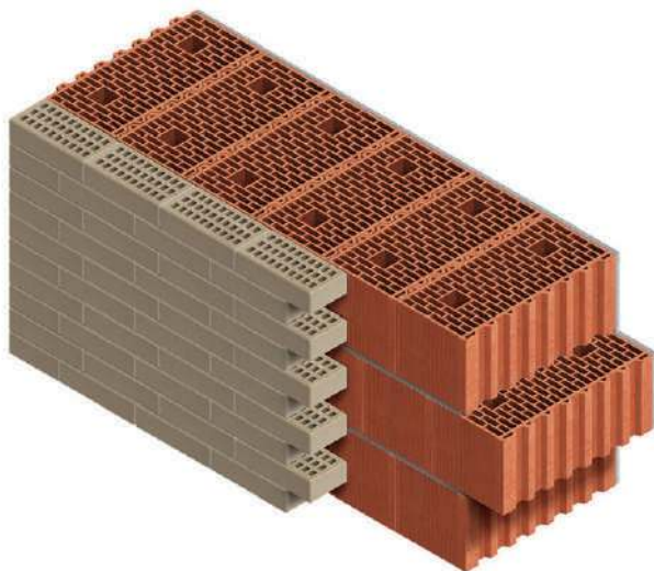
Рис. 2. Конструкция стены из блоков Porotherm 51 и керамического облицовочного кирпича
