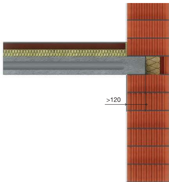
Рис. 13. Опираение плит перекрытия на кладку из блоков Porotherm
